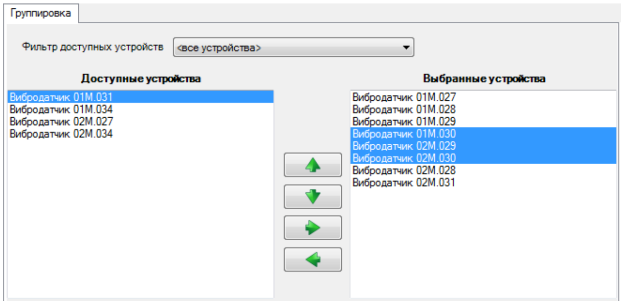
Рис. 6. Фрейм «Группировка»
