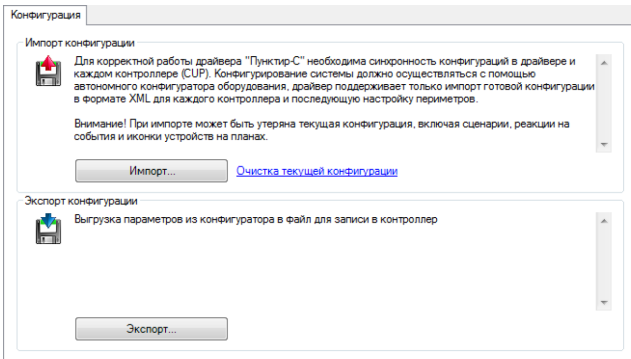
Рис. 3. Фрейм «Конфигурация»
